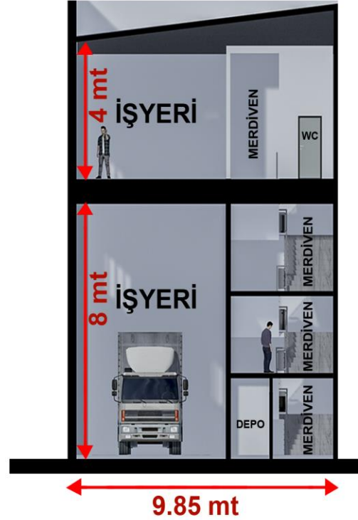
KESİT
