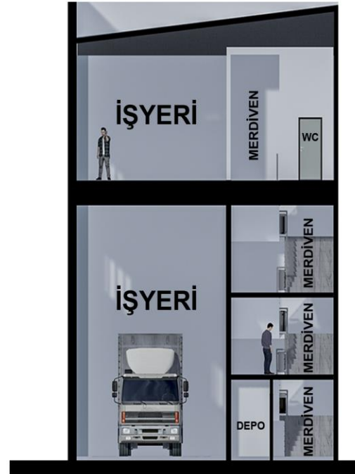
KESİT
